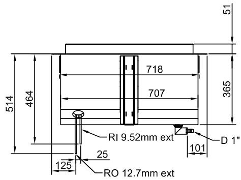
Lato posteriore
